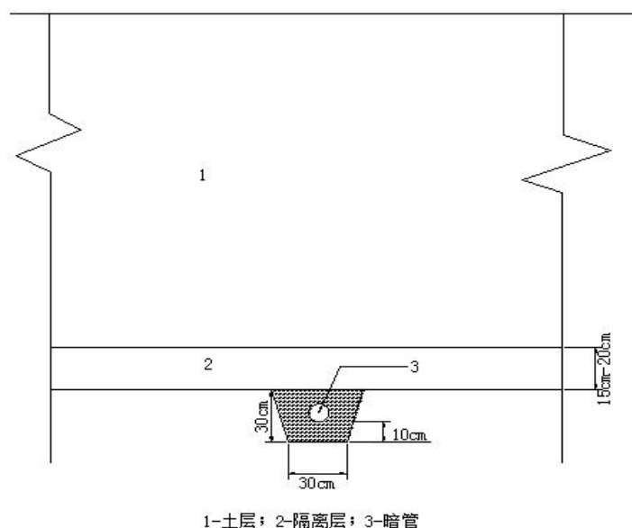
图 2 暗管排盐管道断面示意图
